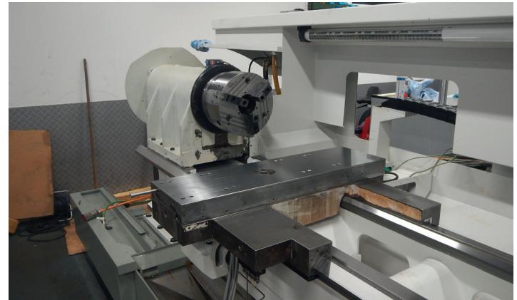
Zyklus CNC Drehmaschine Gildemeister NEF 720 - 2000 (Bild: Maschratur OG)
